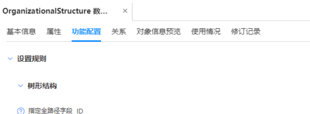
图 9-4 功能配置
