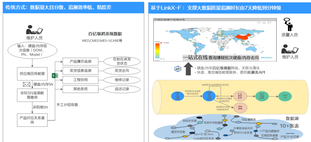
图 12-1 对比优势
