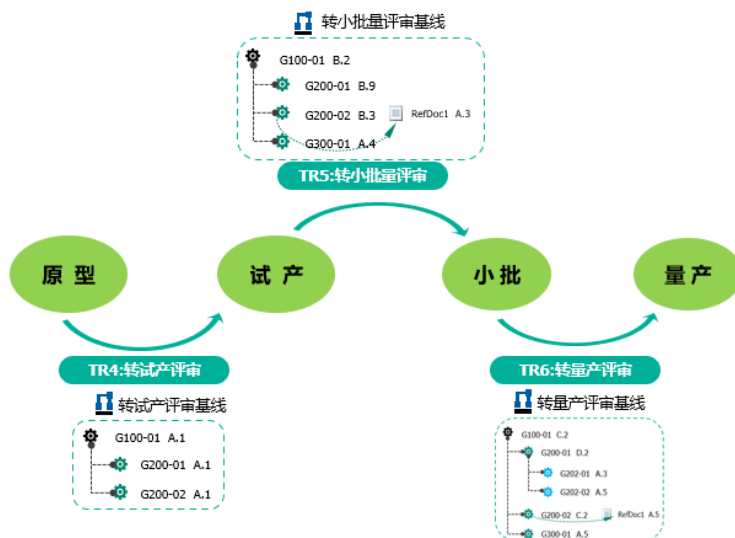
图 10-1 基线
