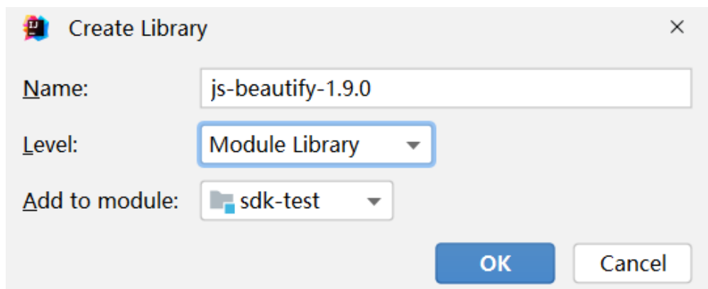
图 2-4 添加 Library
