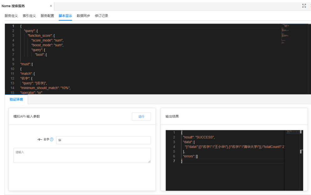
图 4-8 脚本显示
