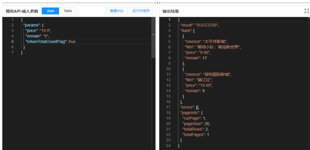
图 5-2 模拟 API
