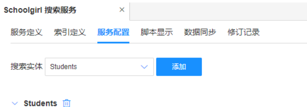
图 4-3 服务配置
