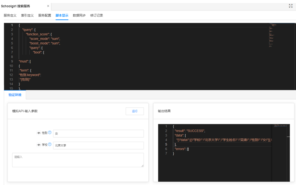
图 4-5 脚本显示
